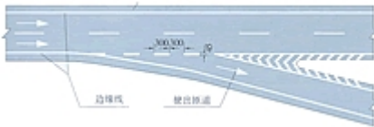
直接式出口标线
