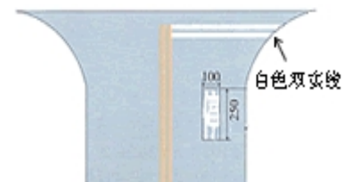
停车让行线（表示车辆在此路口必须停车让干道车辆先行）
